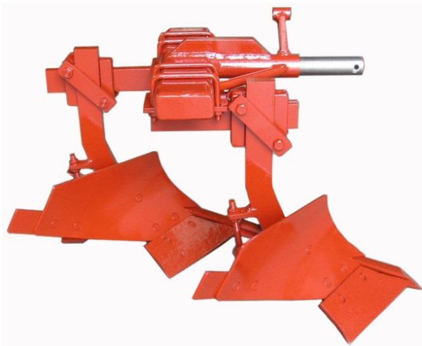
Aratro bivomere 2PV-S Charrue bisoc 2PV-S soc à carcelet Two furrow chisel plough 2PV-S
