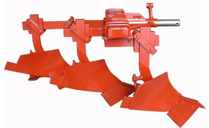
Aratro trivomere 3PV-S con ruotino Charrue trisoc 3PV-S soc à carcelet et roue Three furrow chisel plough 3PV-S with wheel
