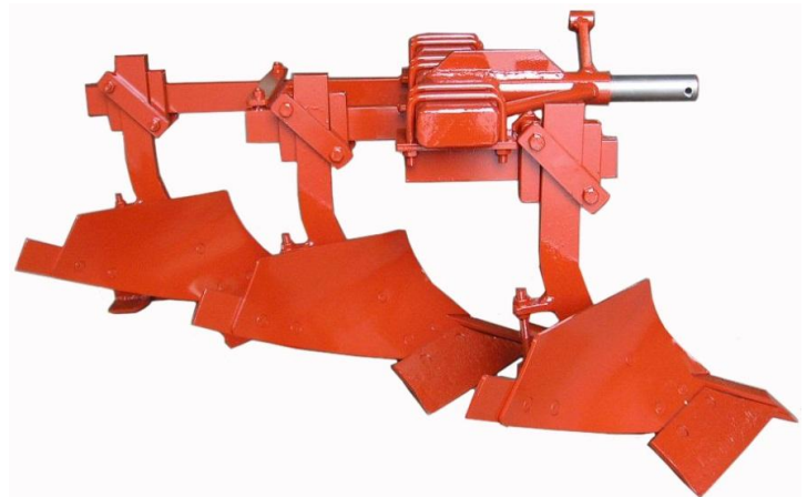
Aratro trivomere 3PV-S con ruotino Charrue trisoc 3PV-S soc à carrelet et roue Three furrow chisel plough 3PV-S with wheel
