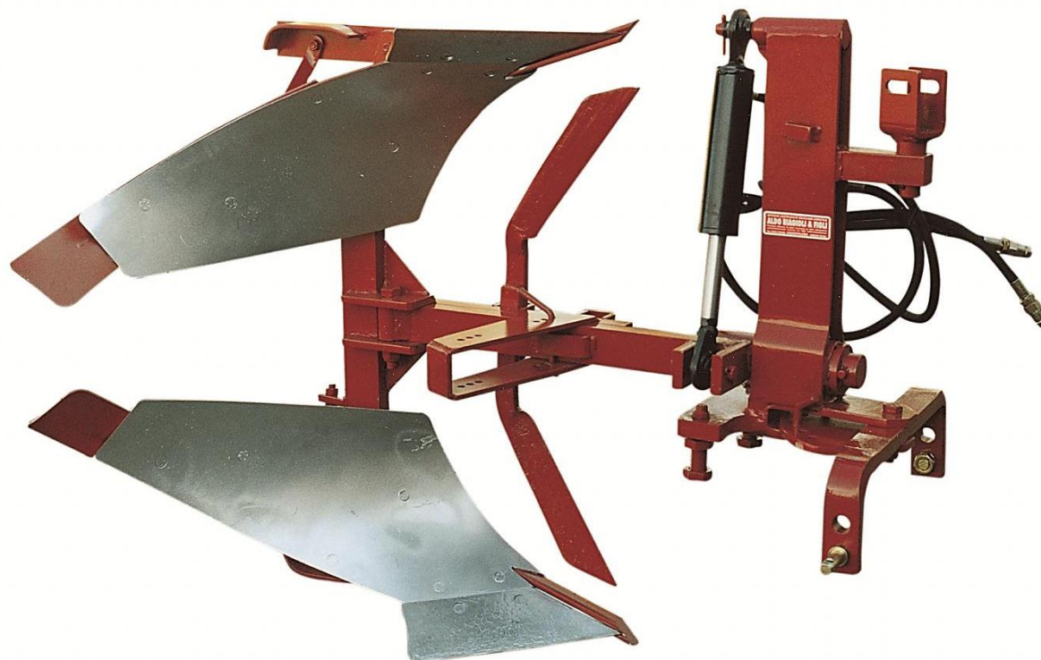
Aratro reversibile VIS ribaltamento idraulico Charrue réversible VIS socs à carcelet retournement hydraulique Reversible chisel plough VIS – hydraulic turnover
